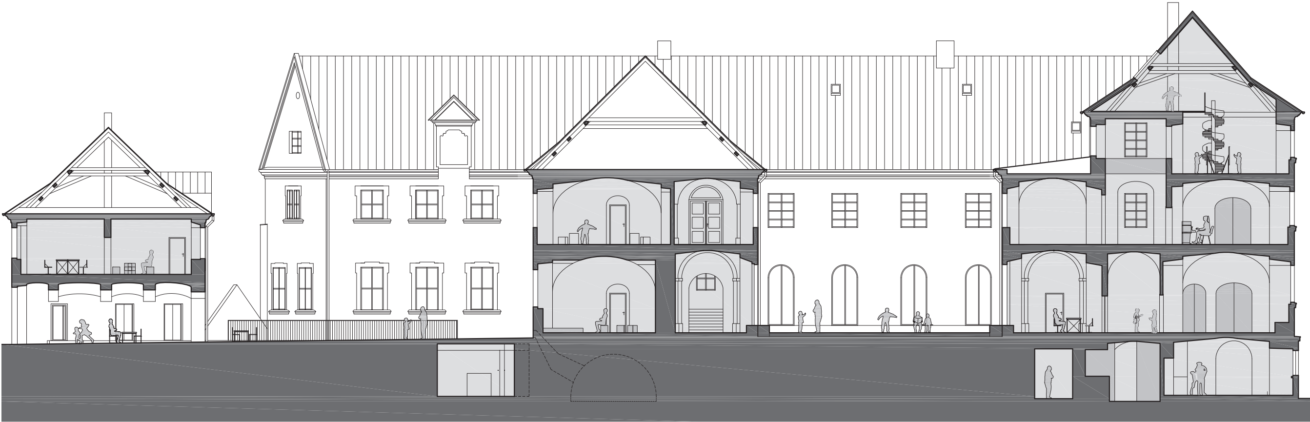
řez A-A'
